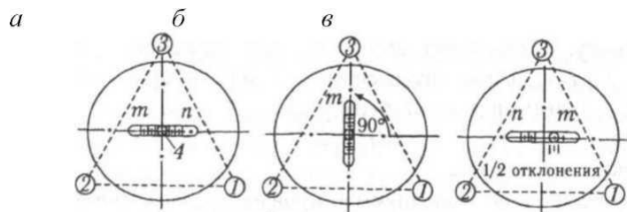
Рис. 2. Проверки цилиндрического уровня: а — установка по двум винтам; б — установка по третьему винту; в — проверка правильности установки уровня; n — оцифрованный штрих лимба; m — число делений микроскопа; 1,2,3 — винты; 4 — пузырек ампулы
